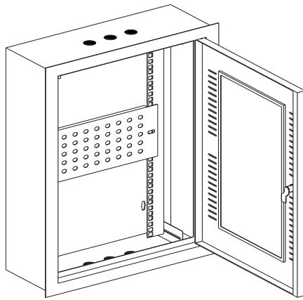
CABINET- 12U 450(W)x150(D)
